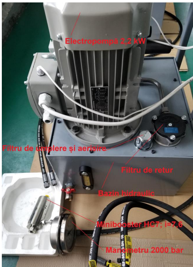
Fig. 2: Modul pompare înaltă presiune: MP3; 2,2 kW; i=7,6 / MPIP-HP1-4,3-HC7-7.6-0.0.
