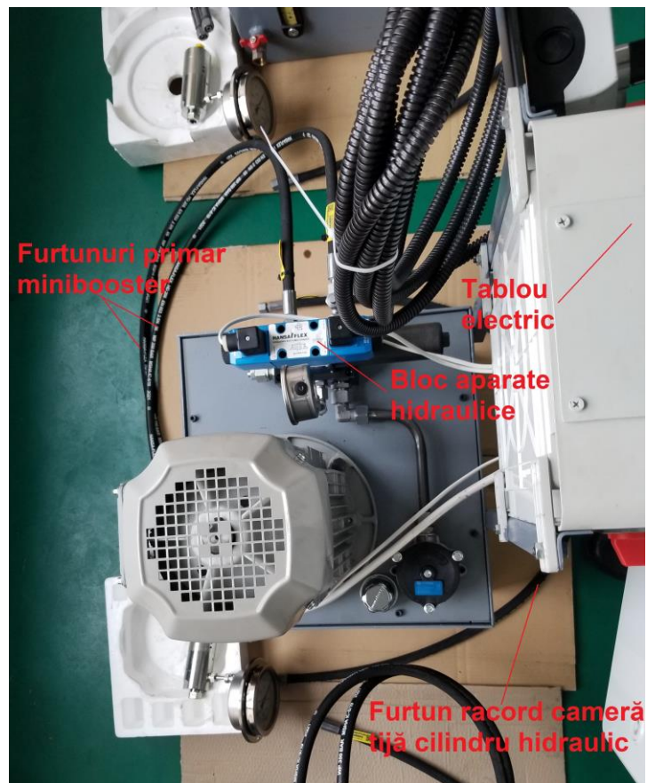
Fig. 2: Modul pompare înaltă presiune: MP3; 2,2 kW; i=7,6 / MPIP-HP1-4,3-HC7-7.6-0.0.
