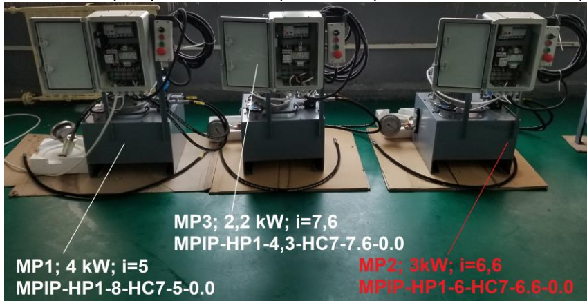
Modulele de pompare executate și montate (tablouri electrice deschise).
