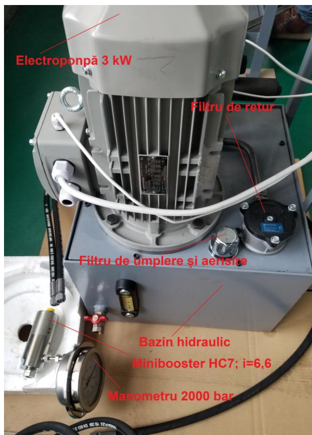
Fig. 2: Modul pompare înaltă presiune: MP2; 3 kW; i=6,6 / MPIP-HP1-6-HC7-6.6-0.0.
