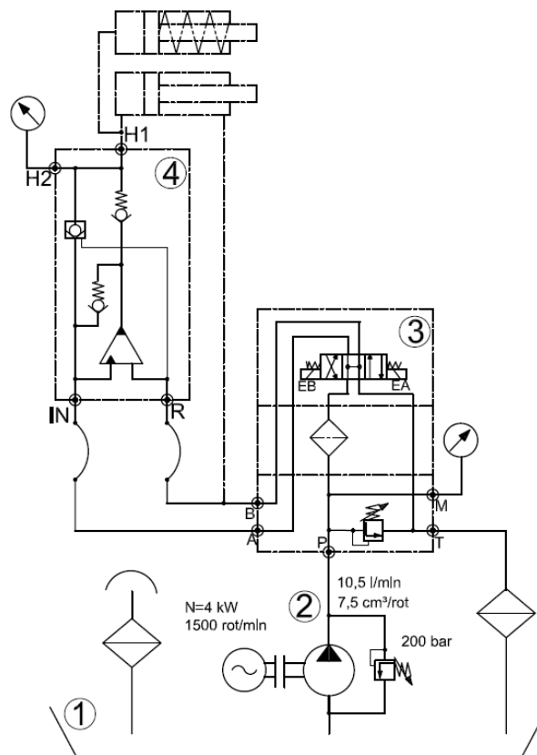
Fig.3: Schema hidraulică a modului de pompare înaltă presiune 1=bazin hidraulic cu filtru retur și filtru de umplere și aerisire; 2=electropompă 4 kW; 3= bloc cu aparate hidraulice; 4= minibooster.
