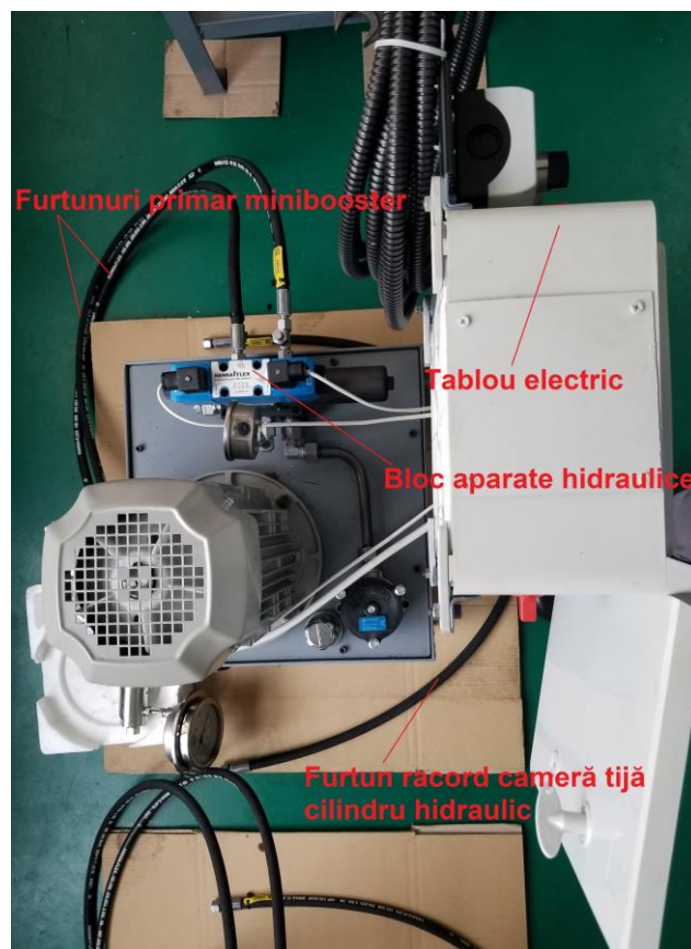
Fig. 2: Modul pompare înaltă presiune: MP2; 3 kW; i=6,6 / MPIP-HP1-6-HC7-6.6-0.0.
