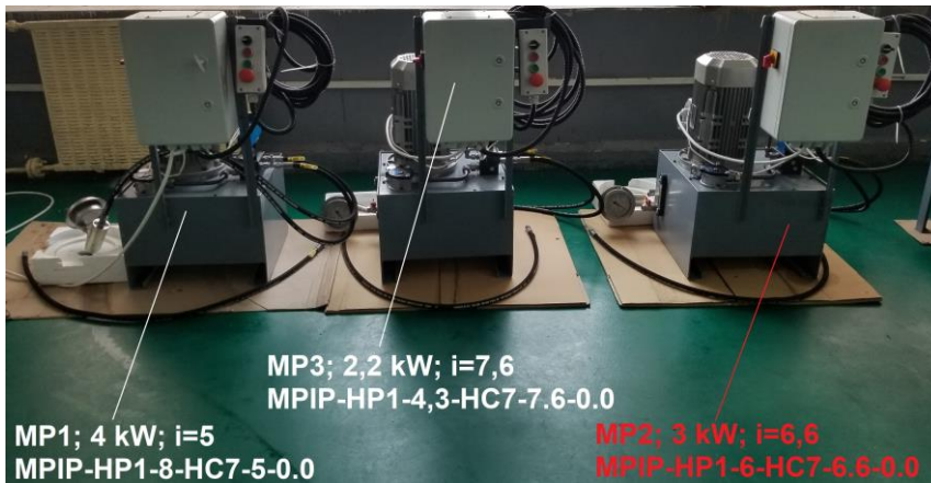
Modulele de pompare executate și montate (tablouri electrice închise).
